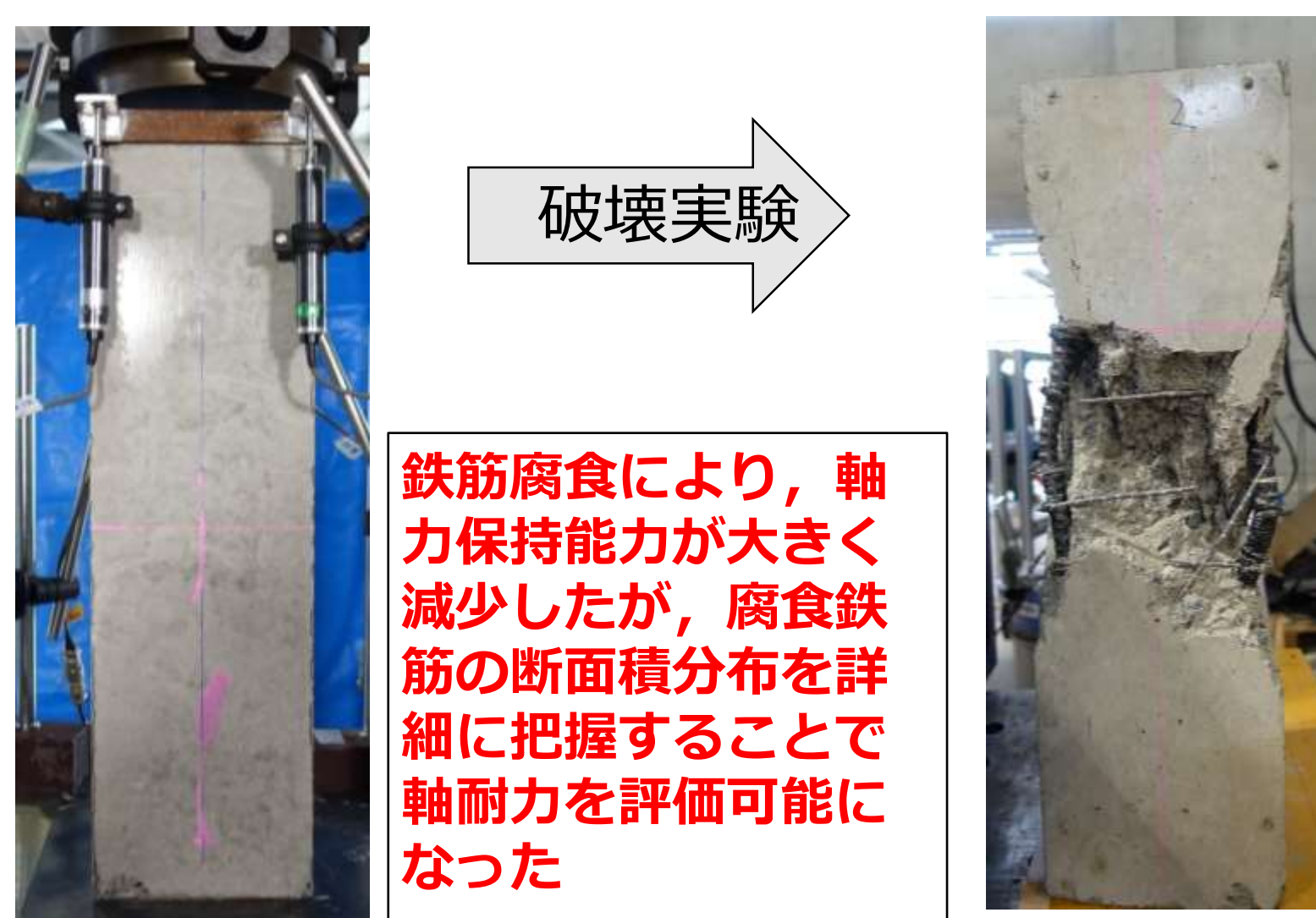
破壊実験による軸耐力評価
