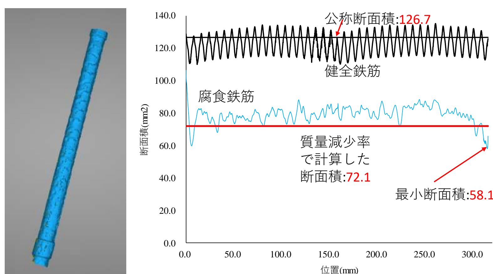
腐食鉄筋の3Dスキャン結果と断面積分布
