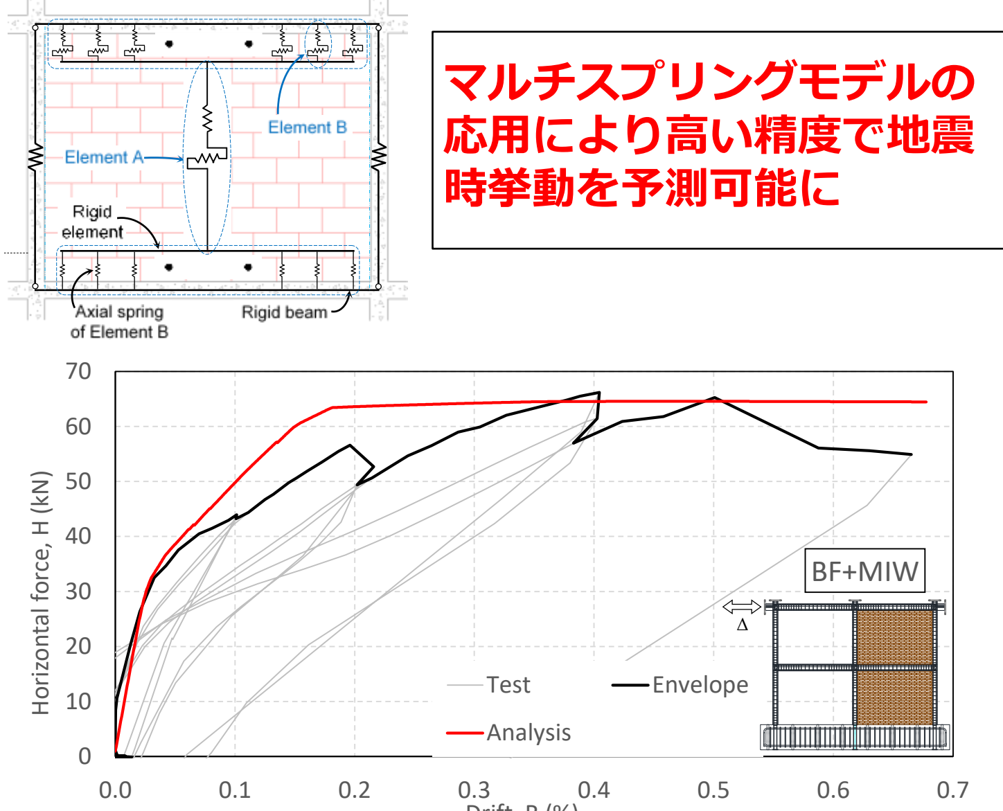
モデル化のコンセプトと実験結果との比較
