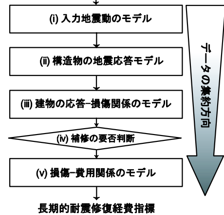
図-1 耐震修復経費指標算出過程
