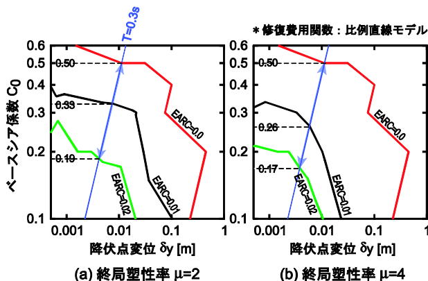
図 - 10 要求スペクトルの使用例
