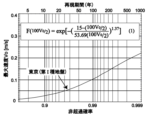
図-2 地震ハザード曲線の例
