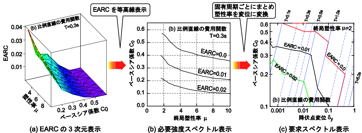
図 - 8 耐震修復経費指標を要求スペクトルに変換する概念図 (地震動シナリオ固定)
