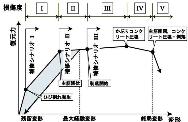
図 - 6 補修シナリオの概念図 2), 6)
