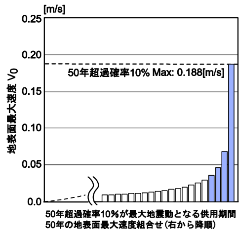
図-3 最大速度の組合せ(降順)推定例
