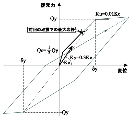
図 - 5 復元力特性
