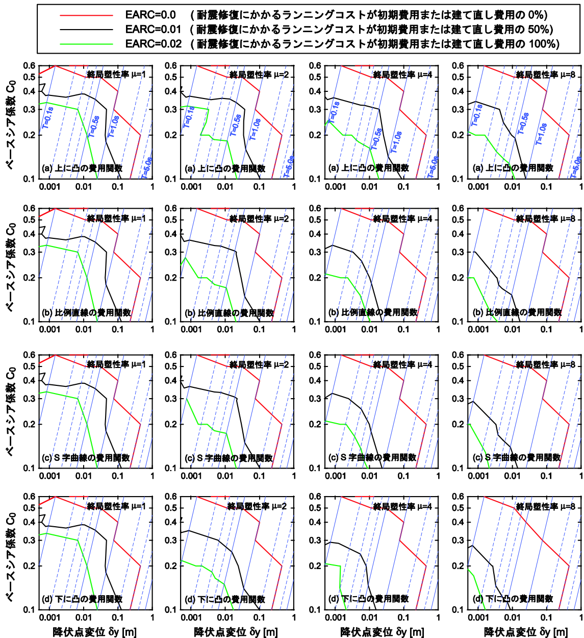
図 - 9 耐震修復経費指標に基づく要求スペクトル表示例
